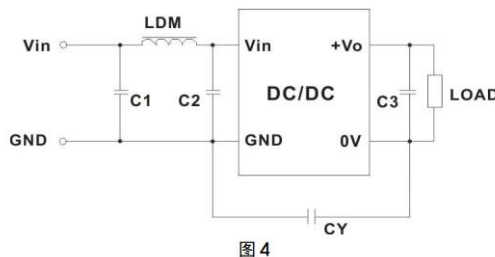
EMC 推荐电路参数值表 (表 2)
